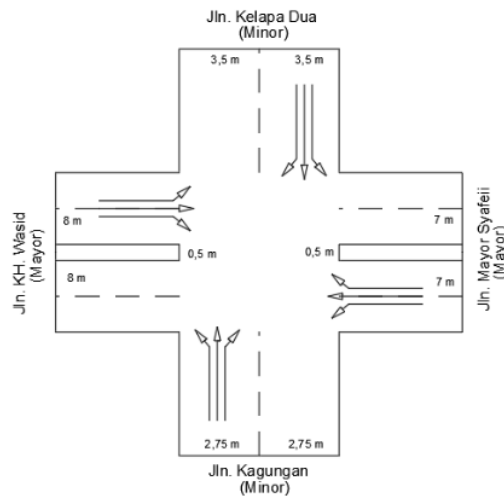
Gambar 1. Penampang Simpang Lontar Sumur Bor
