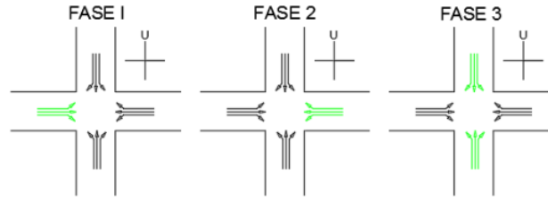
Gambar 2. Pengaturan fase Simpang Lontar Sumur Bor
