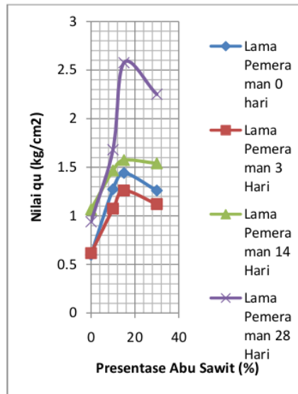
Gambar 5 Grafik Hubungan Nilai qu dengan Presentase Abu Sawit Sumber : Analisis Penulis, 2015
