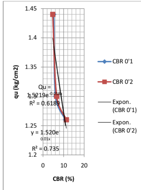
Gambar 9 Grafik Hubungan Nilai qu dengan CBR
