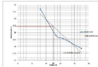
Gambar 2 Grafik Hubungan Kadar Air dengan Jumlah Pukulan
