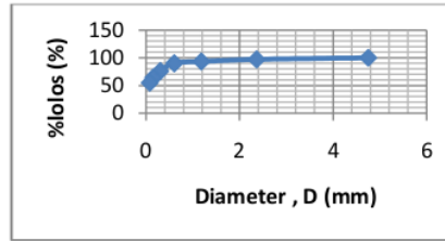
Gambar 1 Grafik Hubungan Berat Lewat Ayakan dengan Diameter Saringan Sumber : Analisis Penulis, 2015
