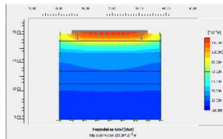
Gambar 20. Hasil Penurunan Total menurut warna Sumber : Hasil analisis, 2016
