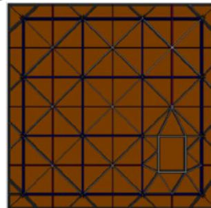
Gambar 4. Tampak Atas Pondasi KSSL Sumber: Hasil Analisa, 2016
