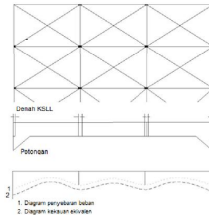
Gambar 2 . Tampak Denah, Potongan dan Diagram Penyebaran Beban dan Kekakuan Ekuivalen pada Pondasi KSSL
