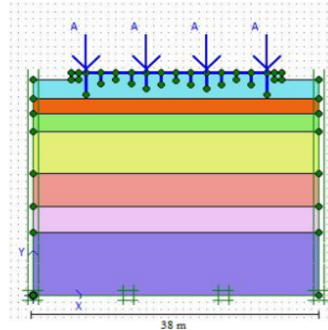
Gambar 18. Pemodelan material Sumber : Hasil analisis, 2016
