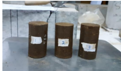
Gambar 6. Benda Uji Kuat Tekan Bebas Sumber: Dokumentasi Penulis, 2019
