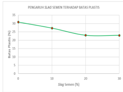
Gambar 9. Pengaruh Slag Semen terhadap Nilai Batas Plastis (PL) Sumber: Hasil Analisa, 2019
