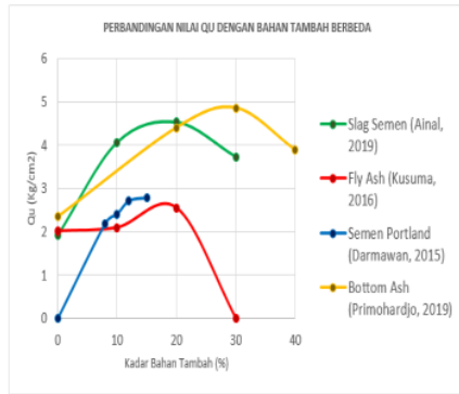
Gambar 17. Perbandingan Nilai Qu terhadap Penelitian Sebelumnya dengan Bahan Tambah Berbeda Sumber: Hasil Analisa, 2019
