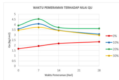
Gambar 12. Pengaruh Waktu Pemeraman terhadap Nilai Qu Sumber: Hasil Analisa, 2019
