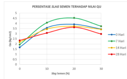
Gambar 11. Pengaruh kadar Slag Semen terhadap Nilai Qu Sumber: Hasil Analisa, 2019
