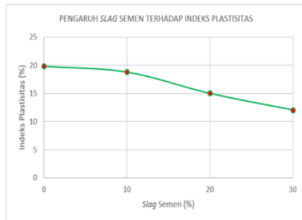
Gambar 10. Pengaruh Slag Semen terhadap Nilai Indeks Plastisitas (PI) Sumber: Hasil Analisa, 2019
