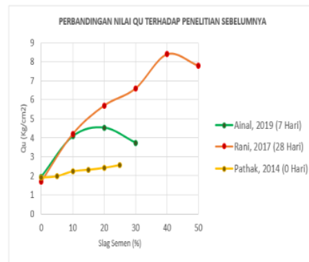
Gambar 16. Perbandingan Nilai Qu terhadap Penelitian Sebelumnya dengan bahan tambah yang sama Sumber: Hasil Analisa, 2019
