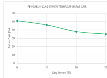
Gambar 8. Pengaruh Slag Semen terhadap Nilai Batas Cair (LL)
