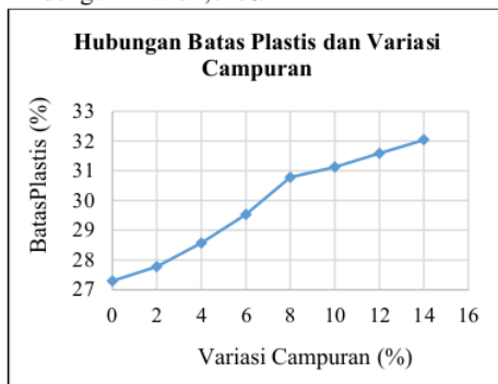
Gambar 5. Grafik Pengujian Batas Plastis Sumber: Analisis Penulis, 2021
