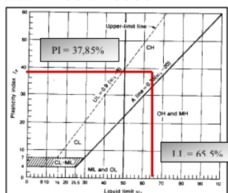
Gambar 2. Grafik Klasifikasi Tanah Sistem USCS
