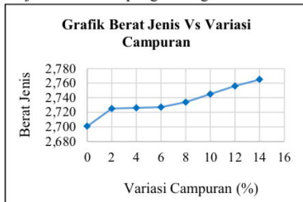
Gambar 3. Grafik Pengujian Berat Jenis Sumber: Analisis Penulis, 2021
