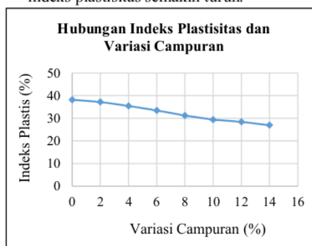
Gambar 6. Grafik Pengujian Indeks Plastis Sumber: Analisis Penulis, 2021
