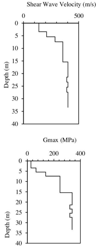
Gambar 4. Profil nilai modulus geser dan kecepatan gelombang geser (Vs) dari program NERA
