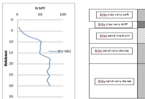
Gambar 2. Profil tanah hasil penyelidikan lapangan untuk BH-062
