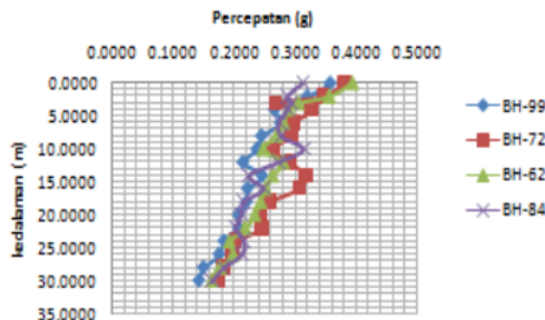
Gambar 8. Profil percepatan di permukaan untuk empat titik untuk mekanisme gempa subduksi
