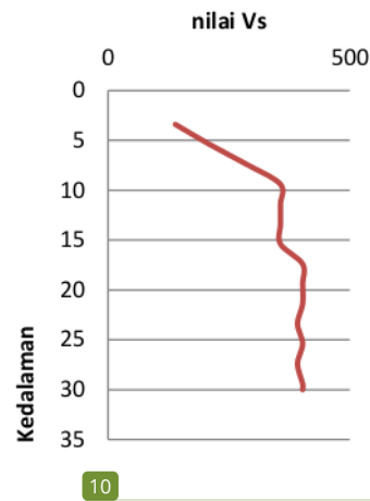
Gambar 3. Profil kecepatan gelombang geser terhadap kedalaman pada BH-62
