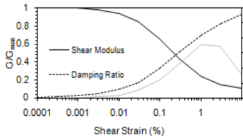
Gambar 5. Hasil perhitungan rasio modulus geser dan damping untuk BH-MF-62
