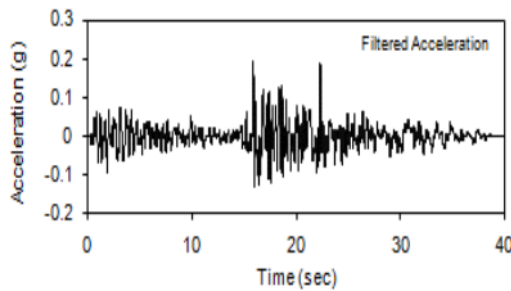
Gambar 6. Ground motion sintetik untuk input NERA
