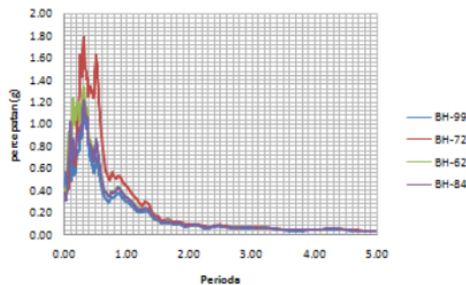
Gambar 9. Respon spektra gempa di permukaan untuk mekanisme gempa subduksi
