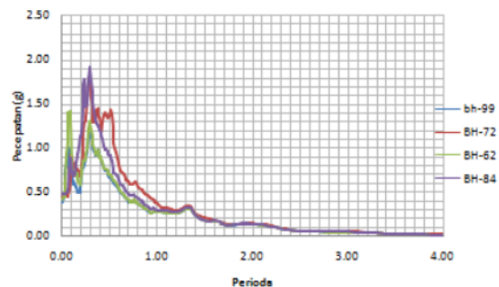
Gambar 11. Respon spektra gempa untuk mekanisme gempa shallow crustal
