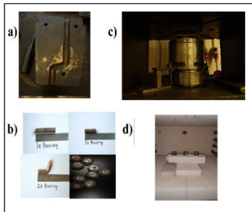
Gambar 1. Tahapan ECAP-parallel channel: a) Cetakan, b) Siklus sampel tekanan, c) Desain cetakan pada mesin press hidrolik, d) Proses perlakuan panas.
