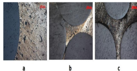
Gambar 5. Struktur mikro perbesaran 100x (a) 1-siklus (b) 2-siklus (c) 3-siklus
