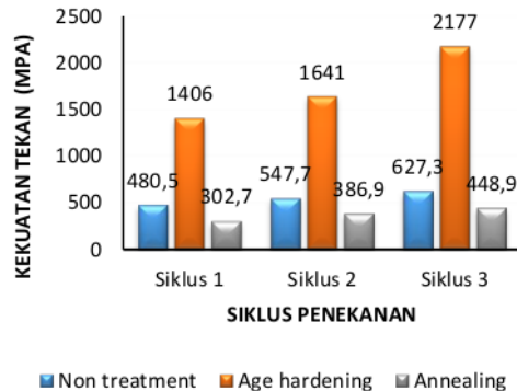
Gambar 4. Grafik hubungan antara siklus penekanan masing-masing treatment terhadap nilai kekuatan tekan.
