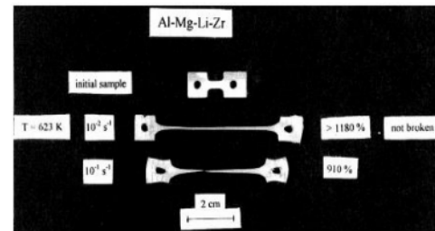
Gambar 2. Superplastisitas laju regangan tinggi dalam paduan yang diproses oleh ECAP sebagai pembanding (Valiev et al. 2016).
