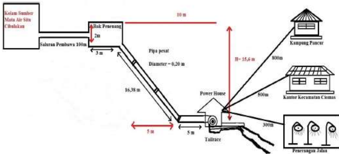
Gambar 3. Model Rancangan PLTMH
