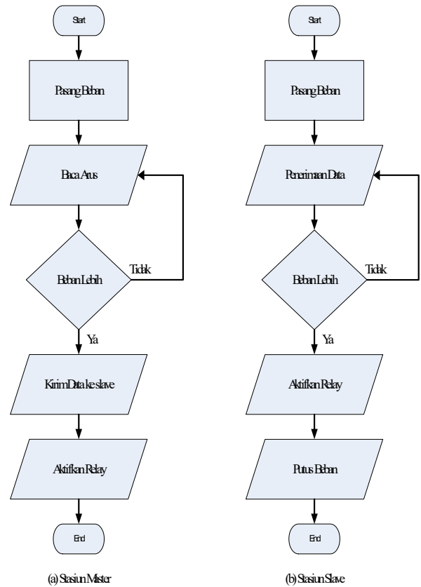
Gambar 6. (a) Diagram Alir Program Stasiun Master (b) Stasiun Slave
