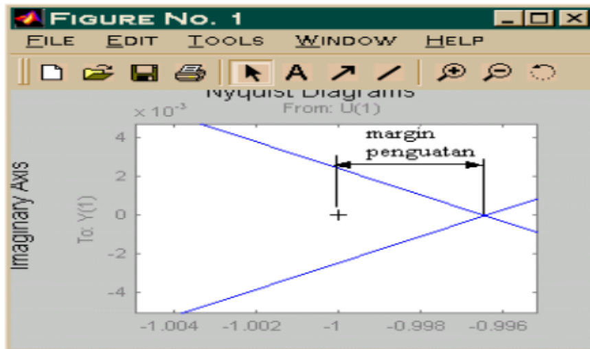
Gambar 9.18 Diagram Nyquist, Diperbesar pada titik -1 + j0
