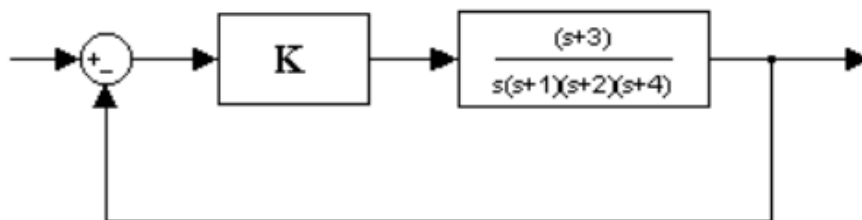
Gambar 7.1 Pengaruh K terhadap Stabilitas
