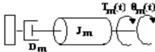
Gambar 5.6 Ekuivalensi Pembebanan Mekanis Pada Motor
