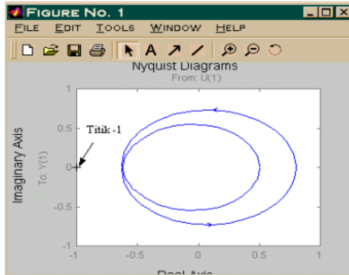
Gambar 9.13 Diagram Nyquist Sistem dengan K=0,5
