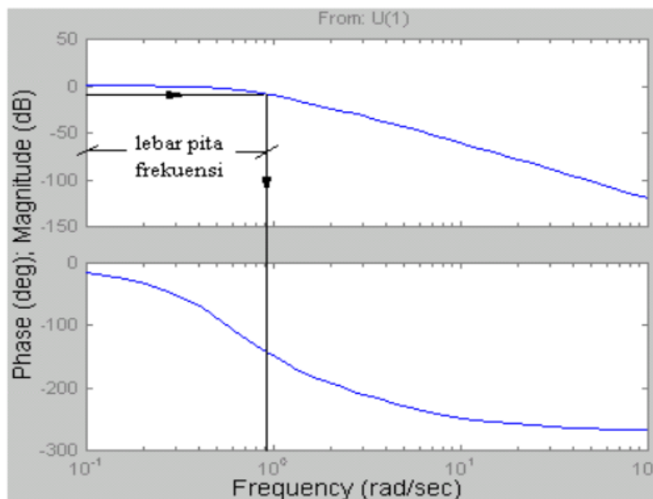
Gambar 9.7 Menentukan Lebar Pita Frekuensi
