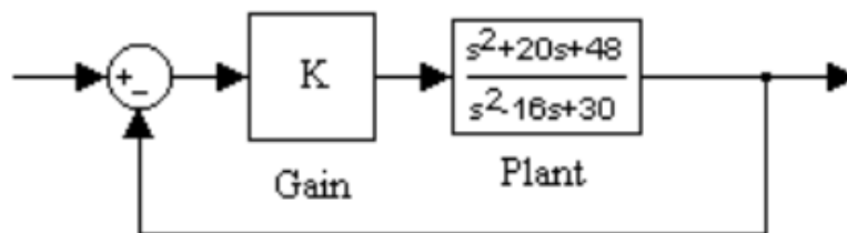
Gambar 9.10 Merancang Sistem Kontrol dengan Diagram Nyquist
