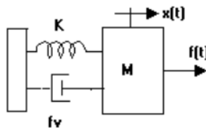
Gambar 5.2 Contoh Sistem Mekanis
