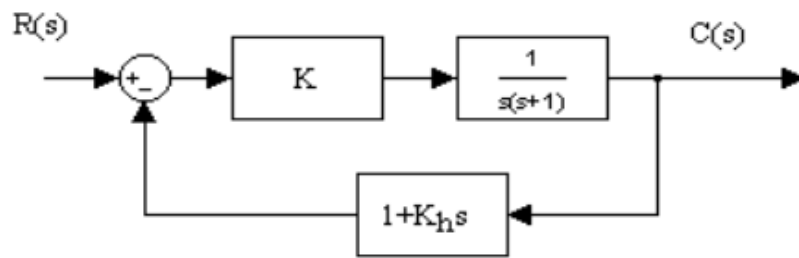
Gambar 7.3 Diagram Blok Sistem Servo Berumpan balik Kecepatan
