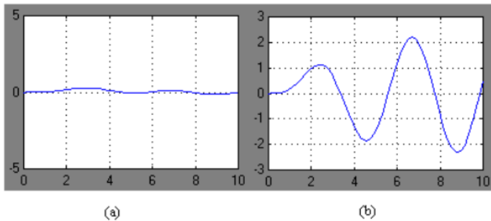
30 Gambar 9.6 Respon Frekuensi Sistem (a). K=1 , (b). K=6
