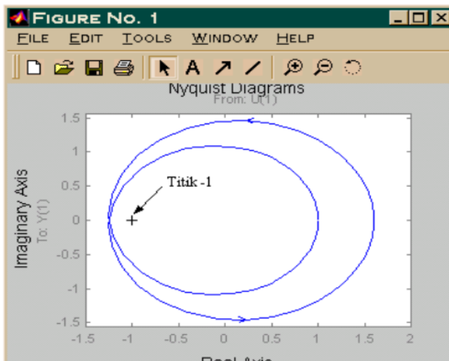
Gambar 9.11 Diagram Nyquist dengan K=1
