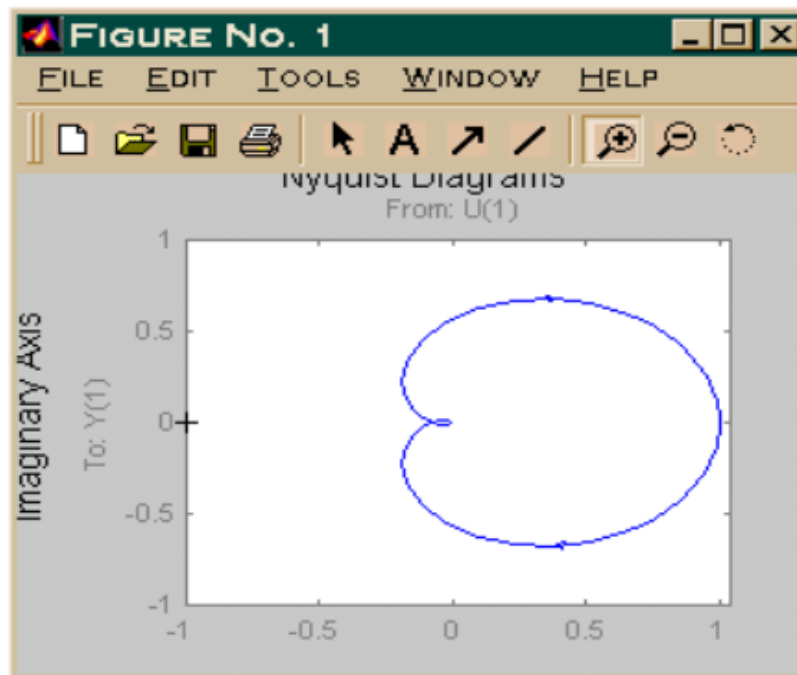
Gambar 9.16 Diagram Nyquist dengan K=10
