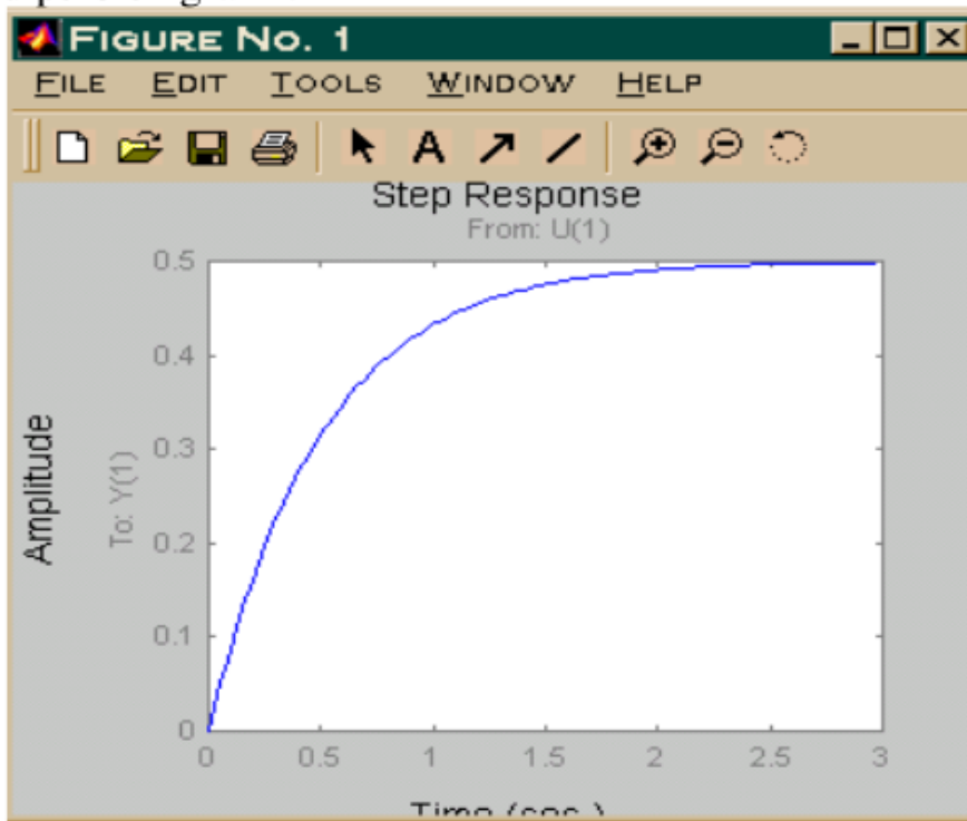
Gambar 6.5 Grafik Respon Sistem 1/(S+1) Lingkaran tertutup
