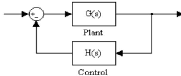
Gambar 9.9 Blok Diagram dengan umpan balik H(s)
