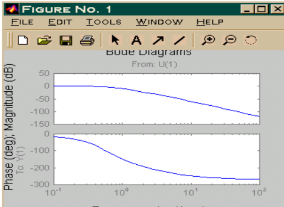
Gambar 9.2 Diagram Bode Sistem Loop Tertutup
