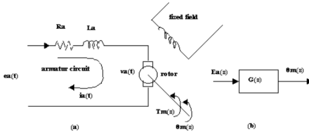
Gambar 5.5 (a). Motor DC, (b). Fungsi Alih
