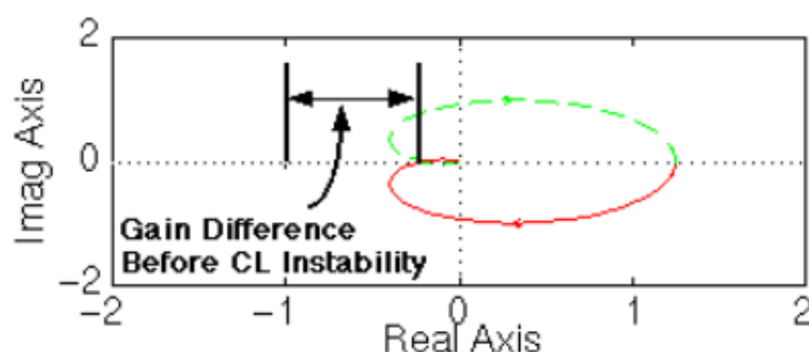
Gambar 9.15 Menentukan Margin Penguatan dengan Diagram Nyquist
