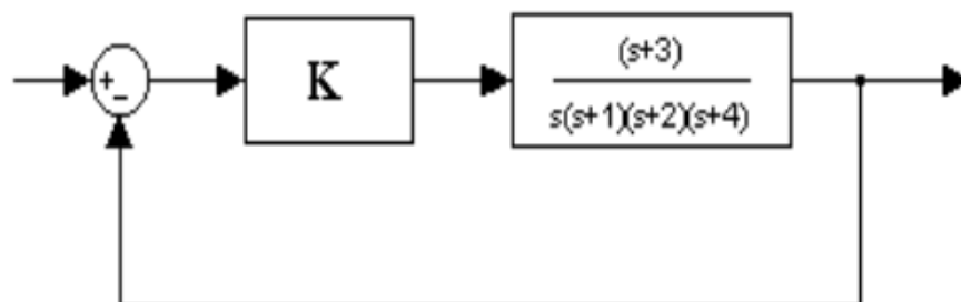
Gambar 4.1 Diagram Blok
