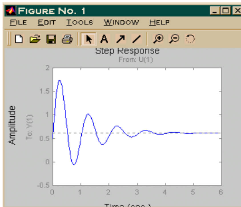
Gambar 9.12 Respon Step Sistem dengan K=1
