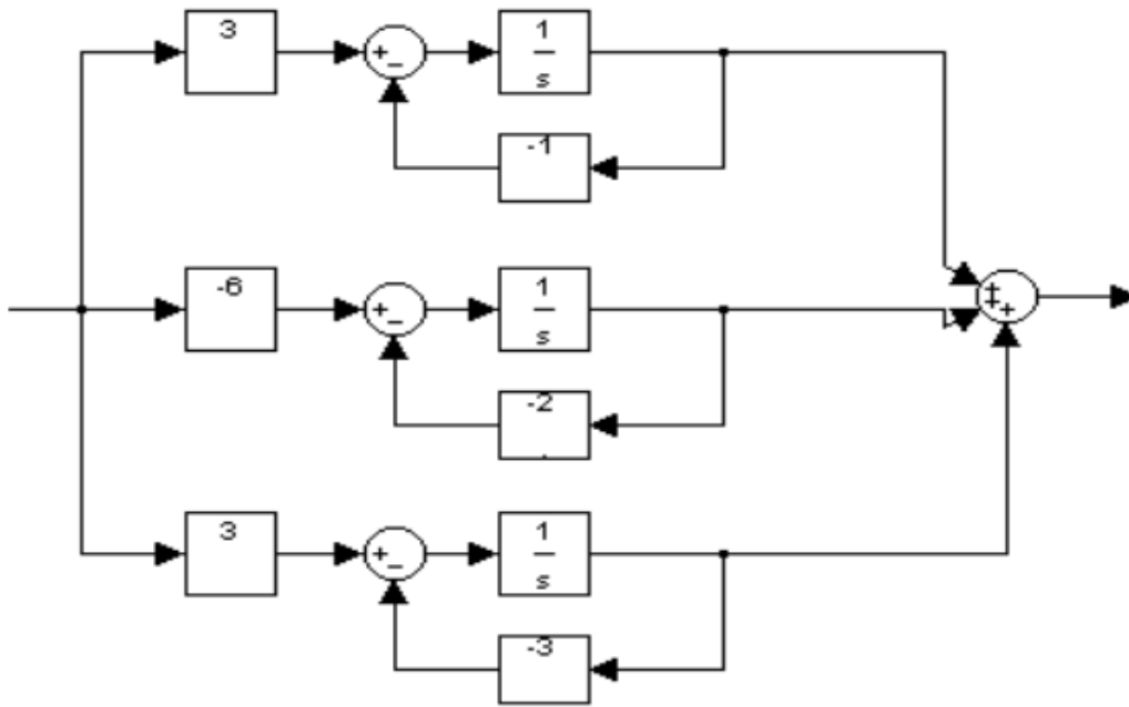
Gambar 10.1 Diagram Blok Sistem dengan Persamaan Keadaan (10.9)
