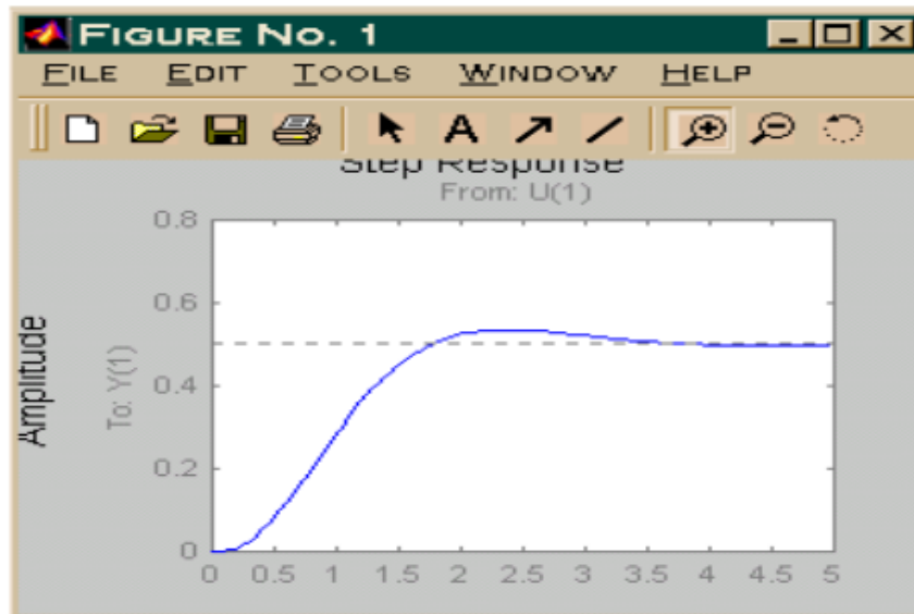
Gambar 9.17 Respon Step Sistem K=10 (stabil)
