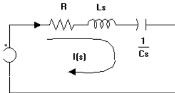
Gambar 5.1 Contoh Sistem Listrik Sederhana
