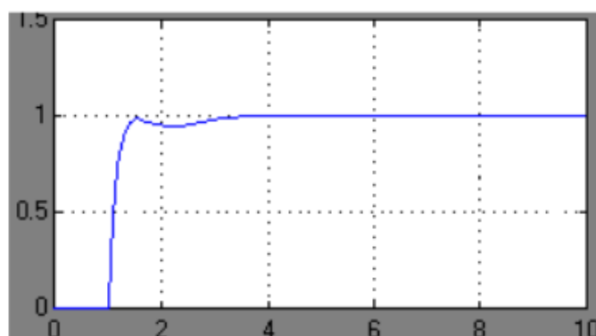
Gambar 8.7 Respon Sistem dengan PID.
