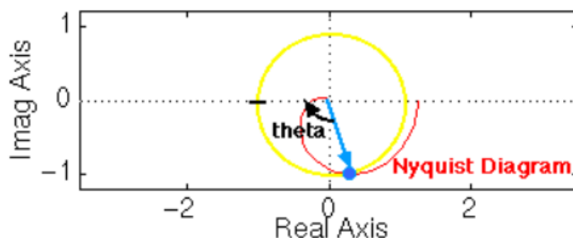
Gambar 9.20 Menentukan Margin Fase
