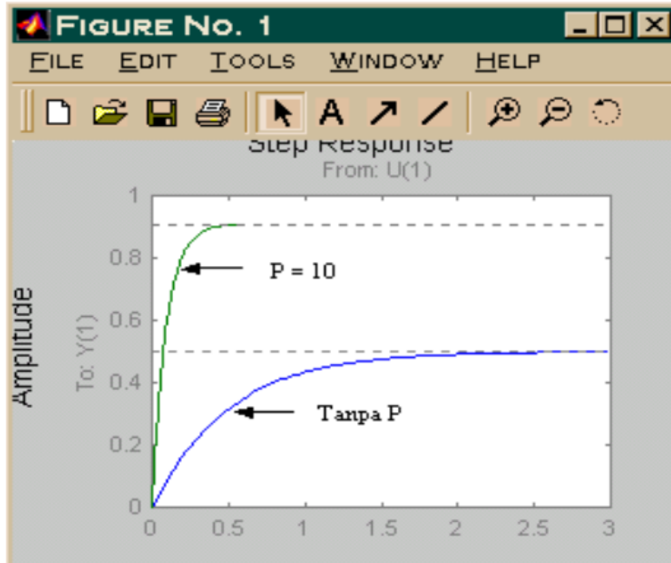
Gambar 8.2 Perbandingan Kontroler P dengan Tanpa Kontroler
