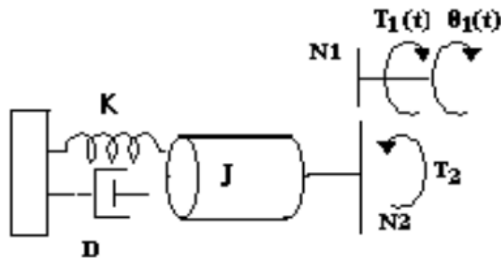
Gambar 5.4 Sistem Rotasi dengan Gir
