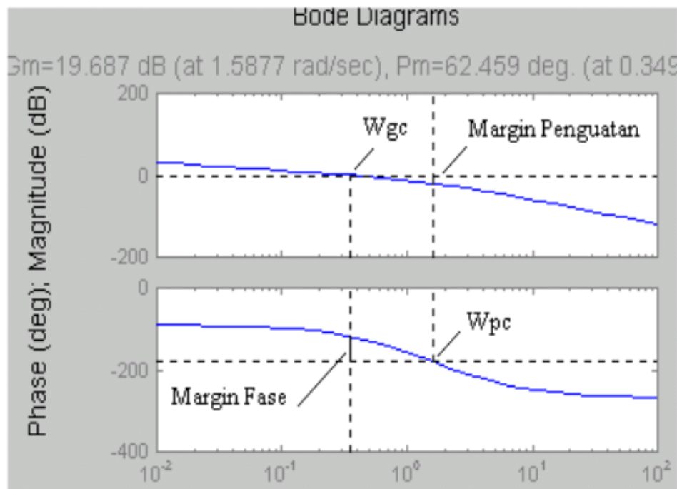
Gambar 9.4 Margin Penguatan dan Margin Fase Sistem.
