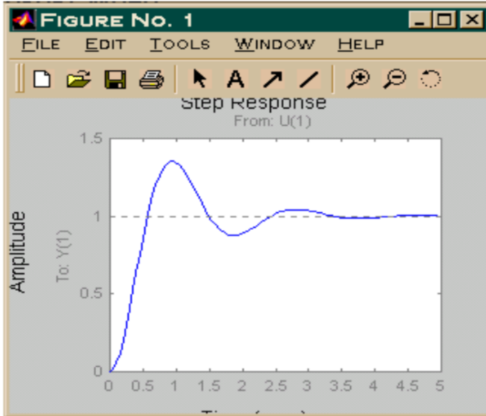
Gambar 7.5 Grafik Step Respon Sistem Servo
