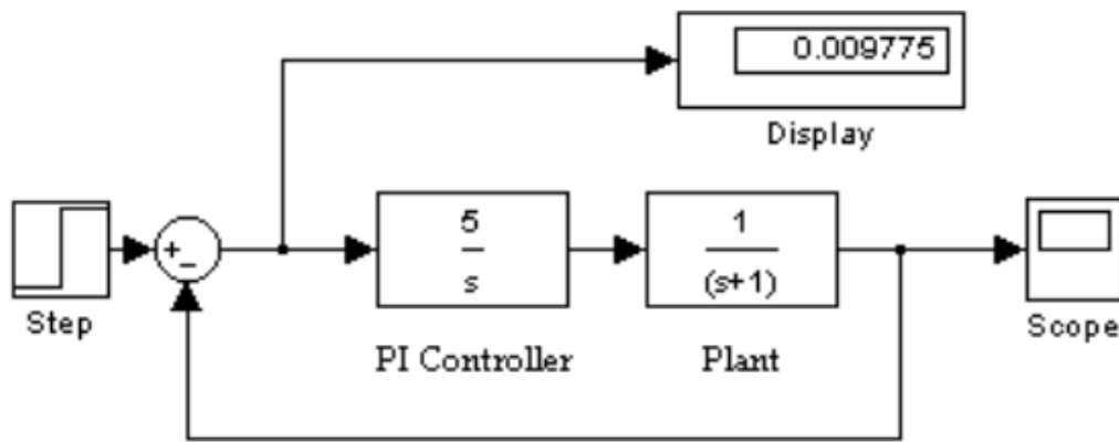
Gambar 8.3 Efek Kontroler PI ( simulasi dengan SIMULINK)
