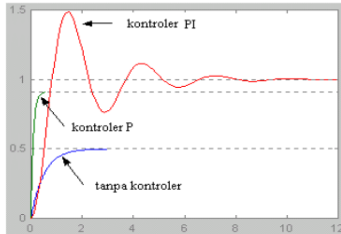
Gambar 8.4 Perbandingan Kontroler PI, P dan Tanpa Kontroler
