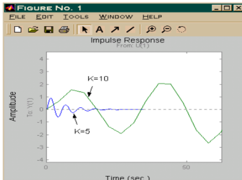
Gambar 6.7 Grafik Respon Sistem dengan K=5 dan K=10
