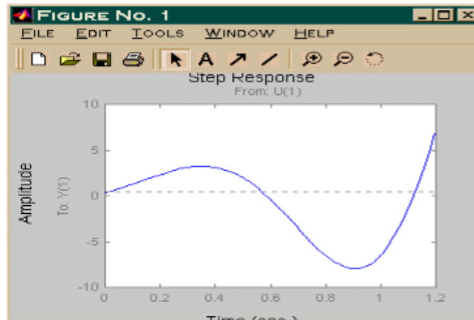
Gambar 9.14 Respon Step Sistem dengan K=0,5
