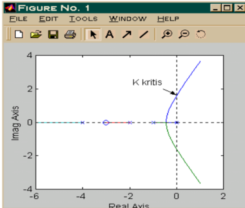
Gambar 7.2 Tempat Kedudukan Akar
