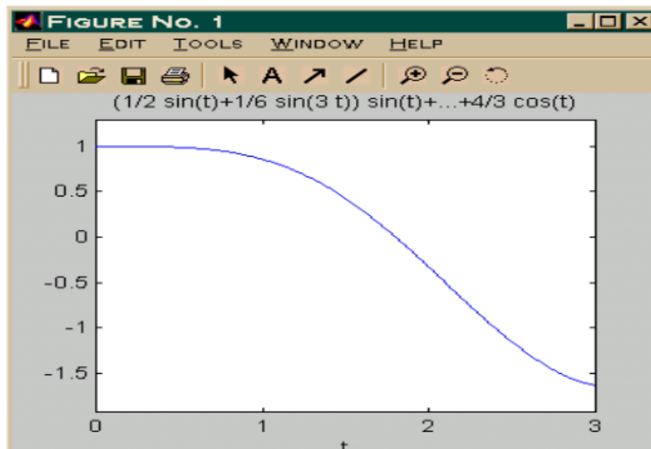
Gambar 3.1 Grafik Persamaan
