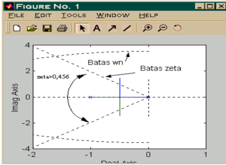
Gambar 7.4 Tempat Kedudukan Akar Sistem Servo
