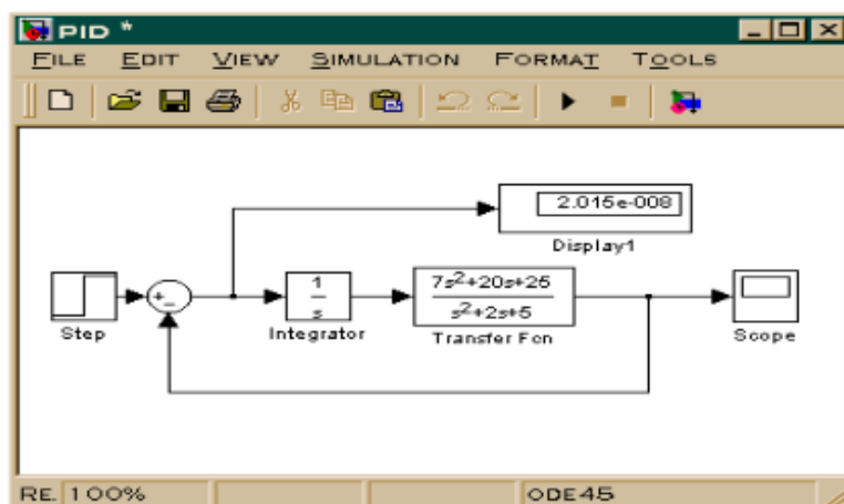
Gambar 8.6 Hasil Perancangan kontroler PID
