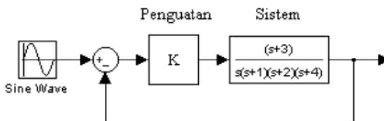
Gambar 9.3 Diagram Blok Sistem dengan Penguat K
