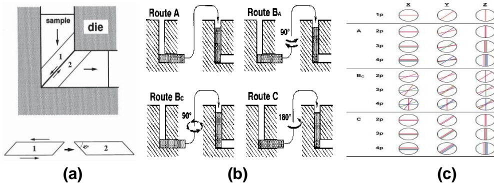
Gambar 3. Mekanisme prosedur regime ECAP a) Desain cetakan yang bekerja gaya tekan jalur 1 dan gaya Tarik jalur 2 b) Route jalur siklus ECAP c) Siklus penekana 2p (pressing) 12x tekan - 4p 4x tekan
