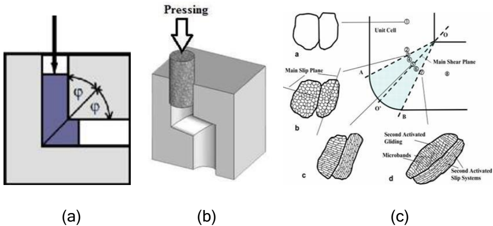
Gambar 4. Tahapan prosedur ECAP: a) pembengkokkan oleh desain cetakan b) Pemberian gaya/tegangan c) proses reaksi yang menghasilkan difusi anar logam
